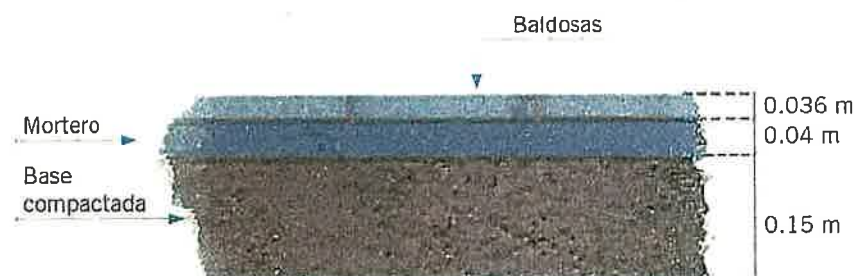
Detalle constructivo pavimento de baldosas. (MINVU, 2017)
